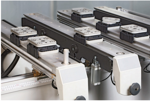
コンソール上に設置される真空クランプブロック (VCBL-K1-140x115x50、VCBL-K1-125x75x50-D-360)
