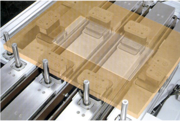
真空クランプブロック VCBL-K2-125x75x100-Q 等を使用したワークの保持
